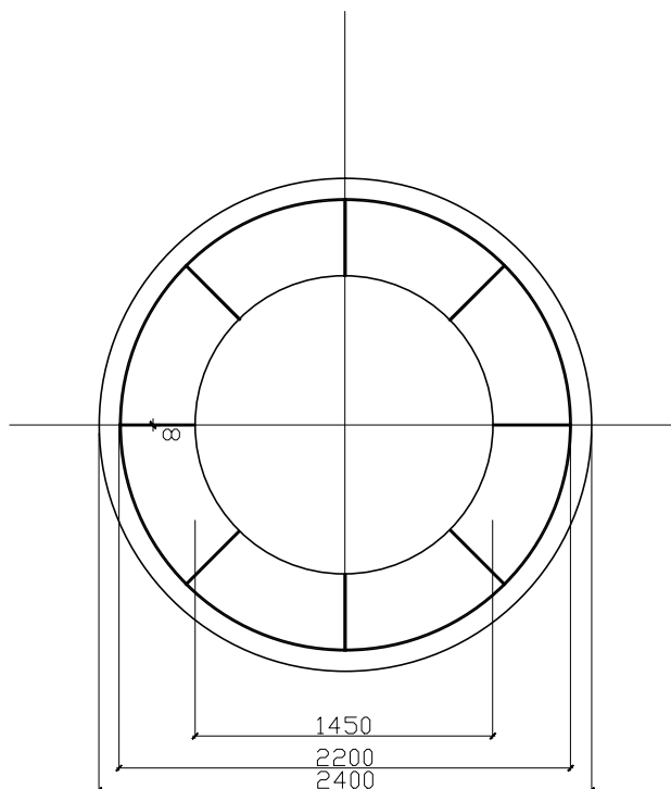
RZUT
