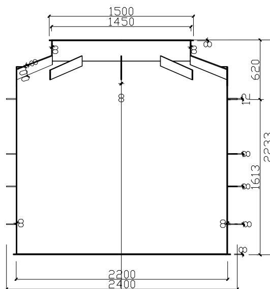
PRZEKRÓJ A-A
