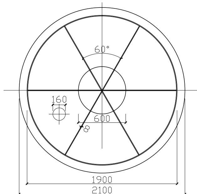
RZUT
