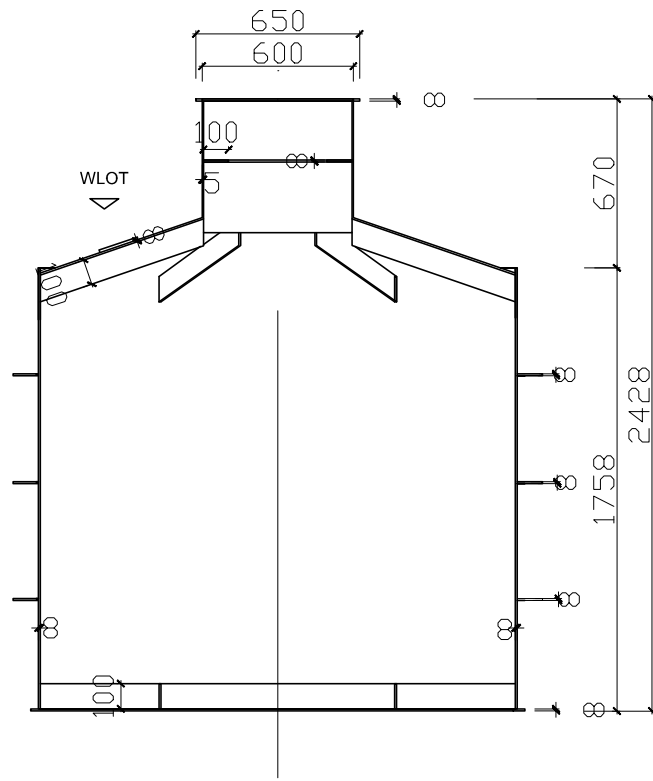
PRZEKRÓJ A-A
