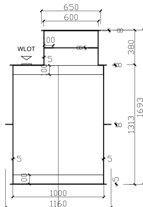
PRZEKRÓJ A-A
