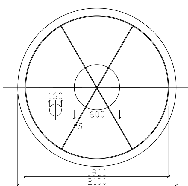
RZUT
