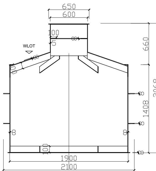
PRZEKRÓJ A-A
