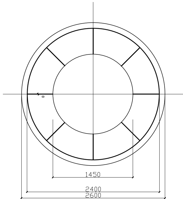
RZUT
