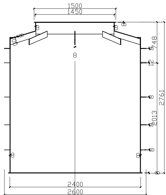
PRZEKRÓJ A-A
