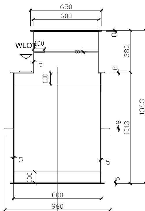
PRZEKRÓJ A-A
