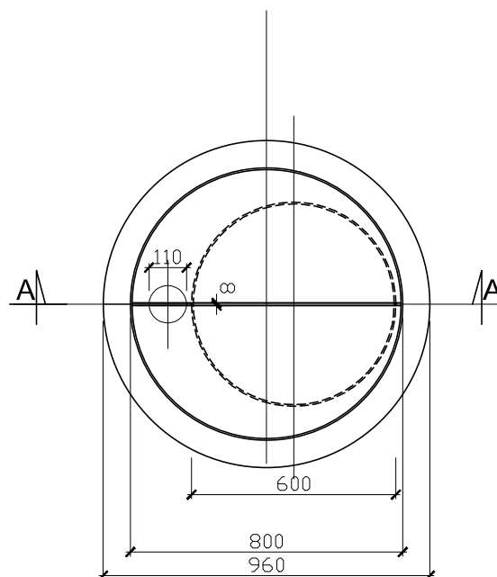
RZUT
