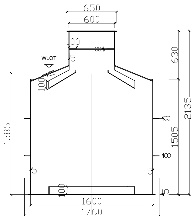
PRZEKRÓJ A-A
