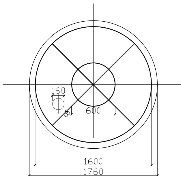
RZUT
