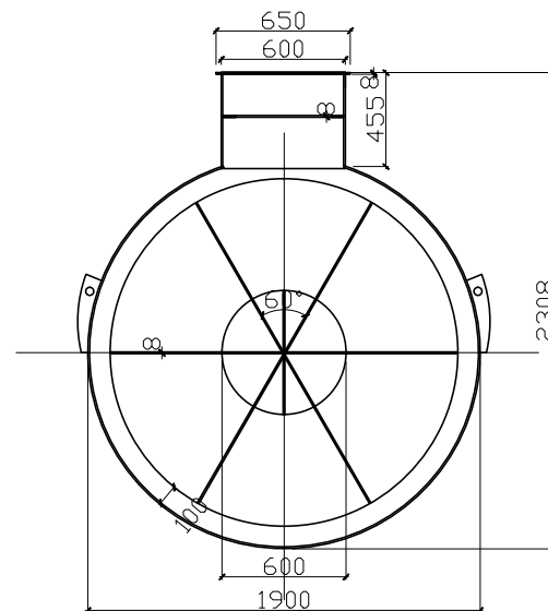
PRZEKRÓJ A-A
